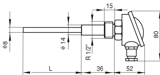
Ugradbene mere elektroprovodne sonde FEL-2
