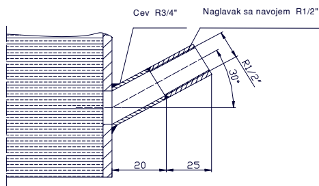
Skica ugradnje elektroprovodne sonde FEL-1
