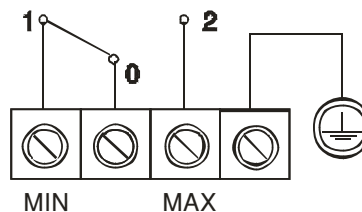
Šema elektropovezivanja
